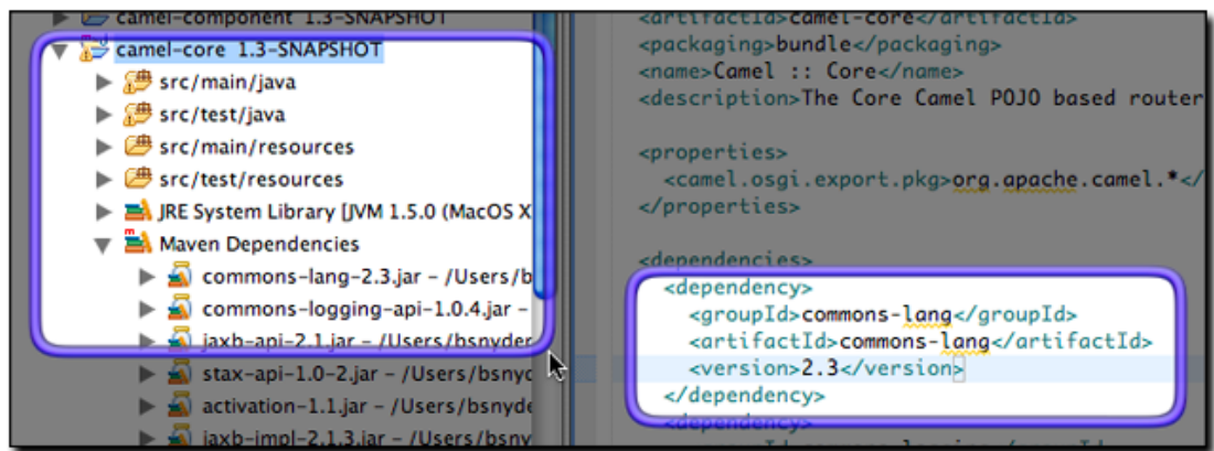
图 14.18. 手动给项目的POM添加一个依赖
