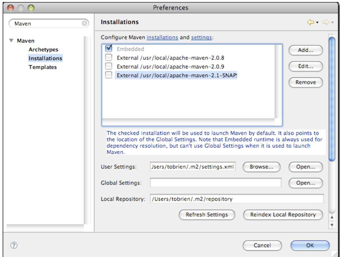
图 14.38. Maven安装选项页面
