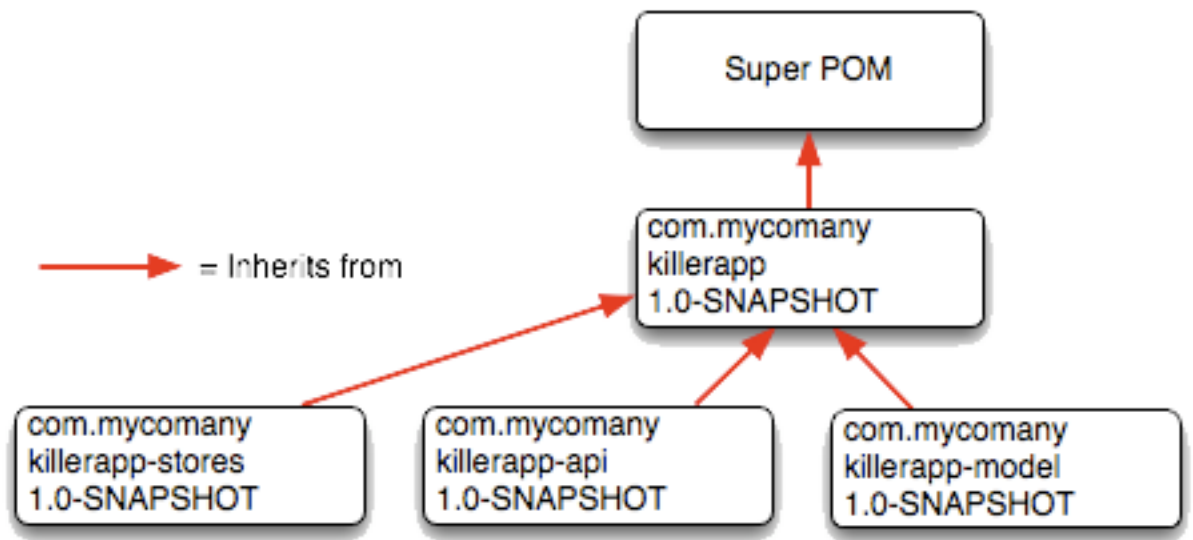
图 9.2. 超级POM永远是最基础的父POM
